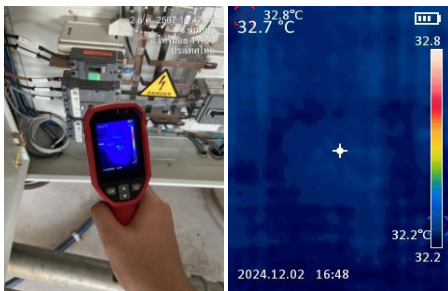
ตรวจสอบความร้อนBreaker inverter 32.7 °C
