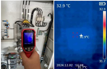
ตรวจสอบความร้อนMCCB 32.9 °C
